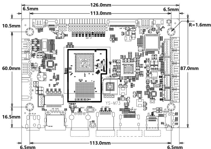
外形尺寸图
