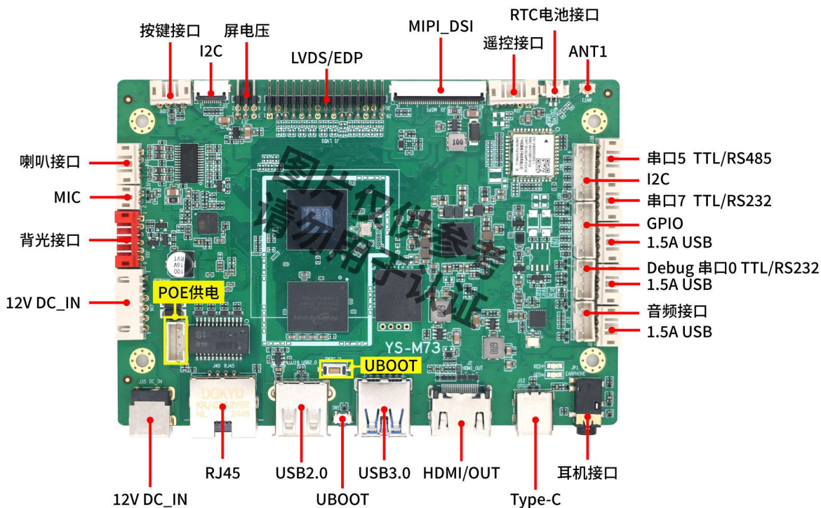
正面接口图
