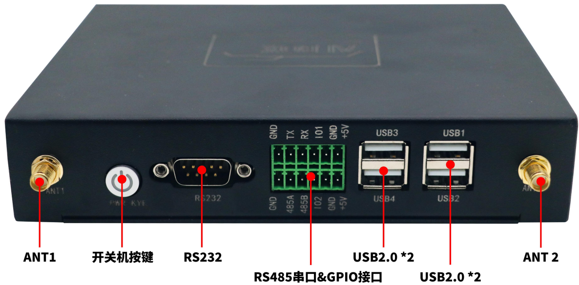
背面图
