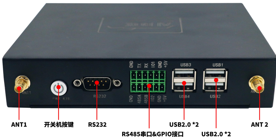
背面图
