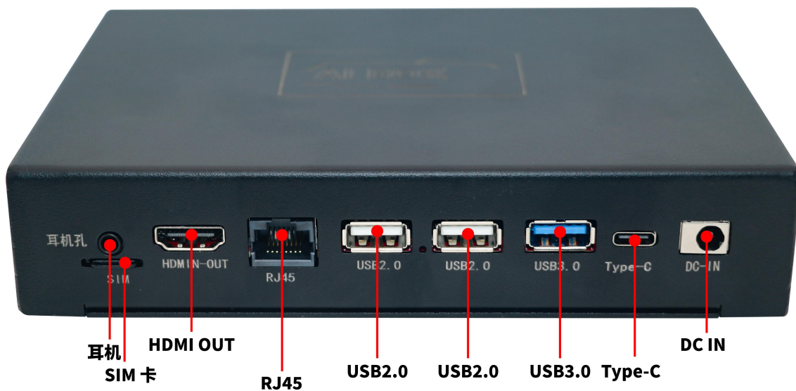
正面图
