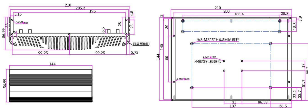
尺寸图
