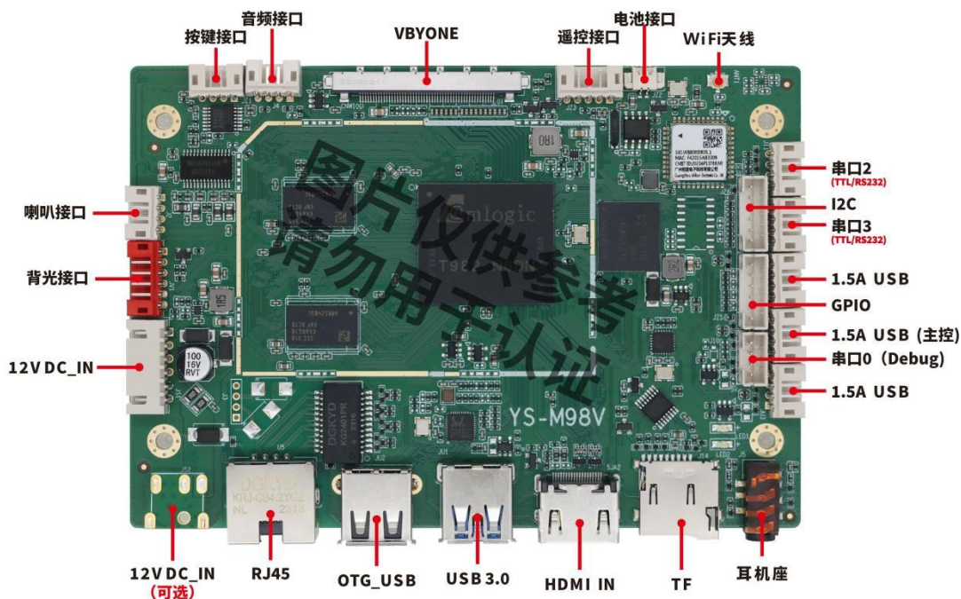
正面接口图
