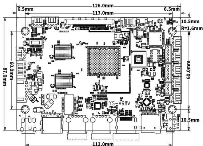
外形尺寸图
